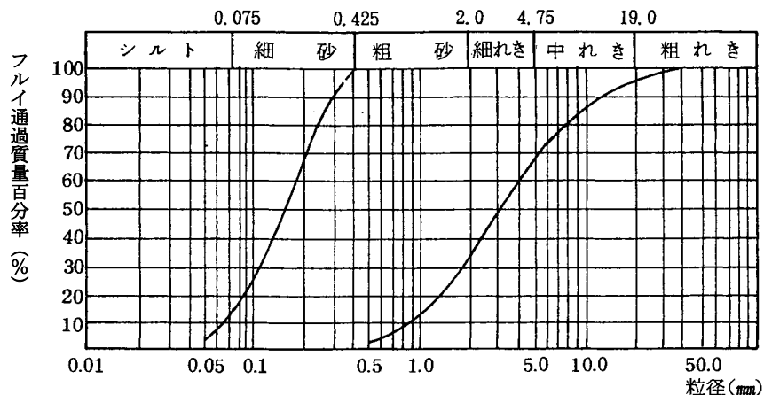
図3-1 使用砂の粒径加積曲線
