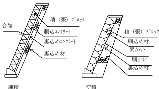
図2-3 コンクリートブロック工
