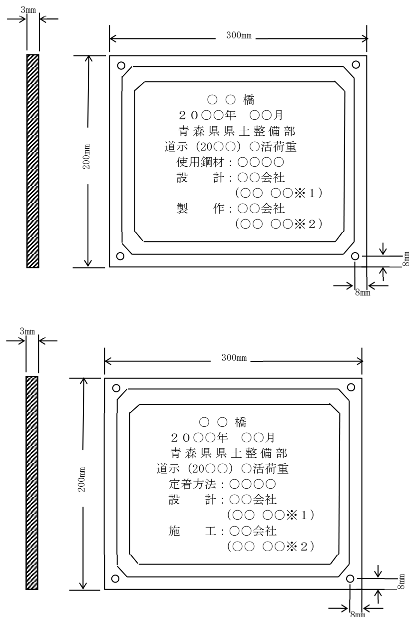
図2-2 橋歴板（アルミニウム）例
