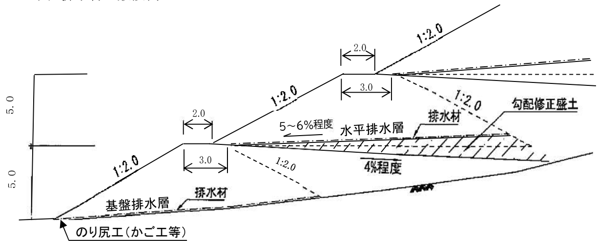
図. 排水材の敷設例
