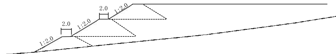
図. 盛土形状の例
