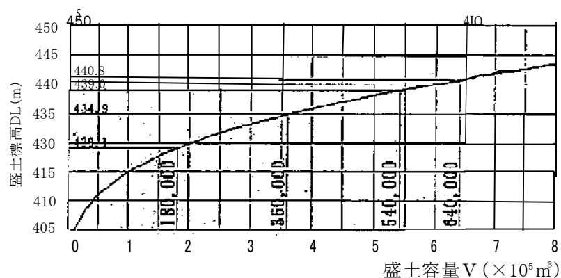
盛土標高～盛土容量関係図
