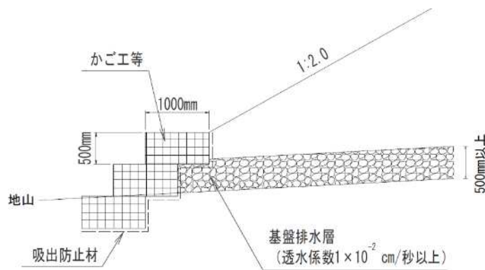
図. 基盤排水層施工図(例)
