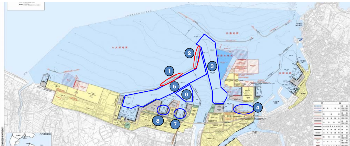
施設配置図
