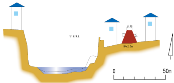
<駅前地区 整備イメージ (横断面図)>
