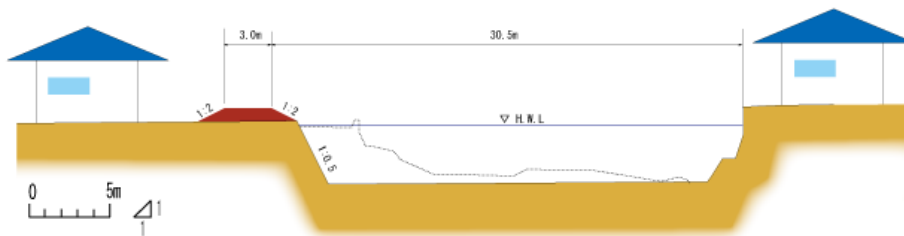
<整備イメージ (横断面図)>
