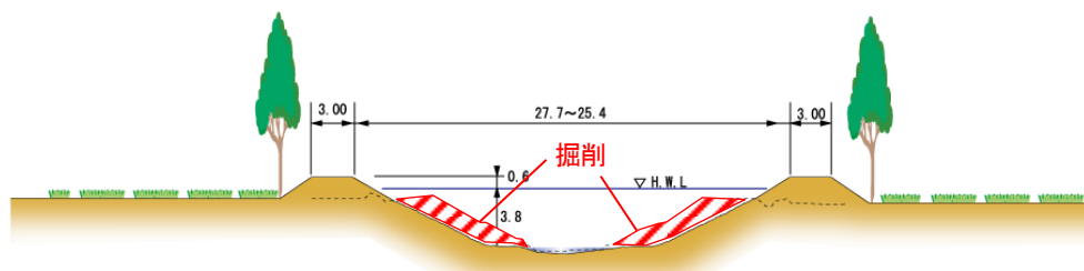
<整備イメージ（横断図）>
