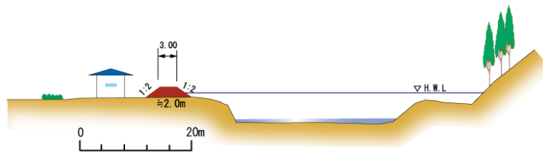
<整備イメージ（横断図）>
