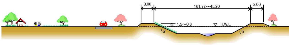
整備イメージ（馬淵川合流点～渡の葉橋の放水路）
