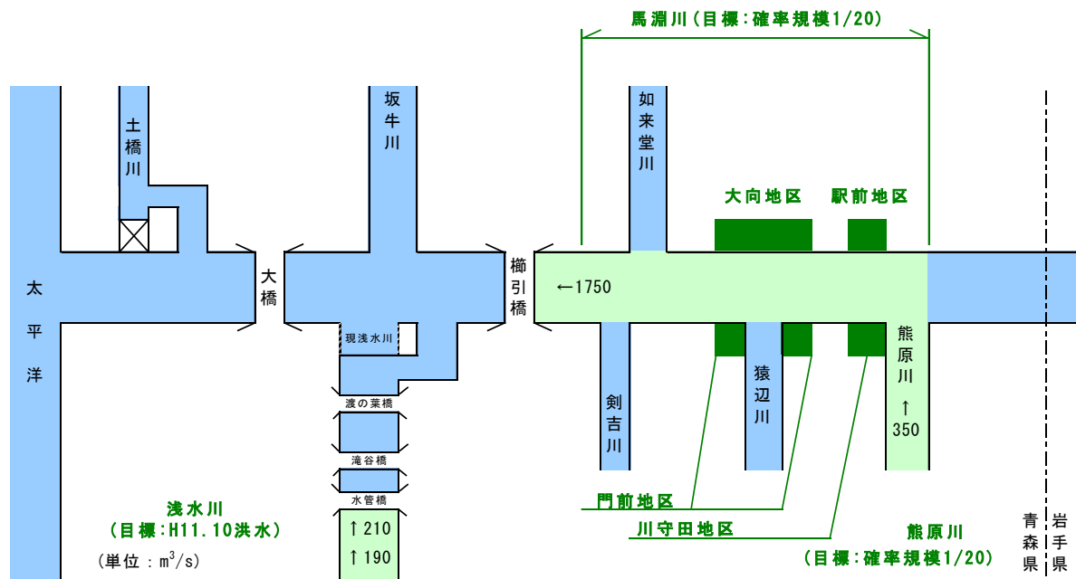
<整備計画目標流量配分図>
