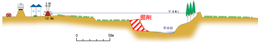
A-A' 相内工区 整備イメージ
