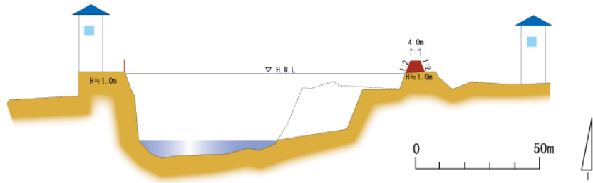
<大向・駅前地区 整備イメージ (横断面図)>
