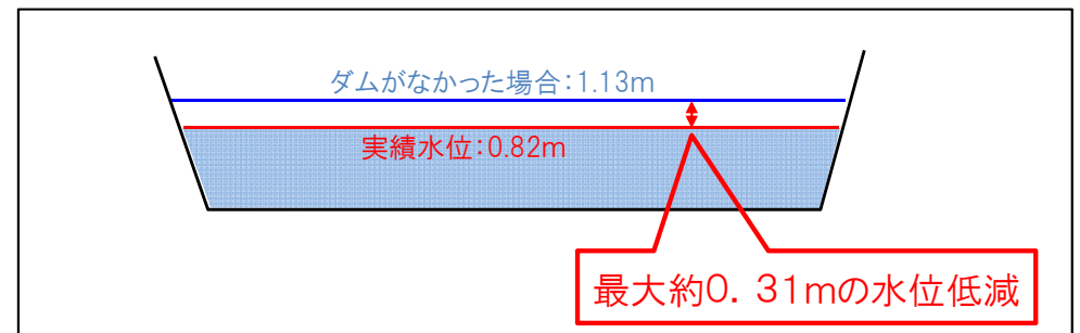
福泉地点での水位低減効果
