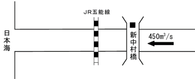
図2-2 整備目標流量配分図
