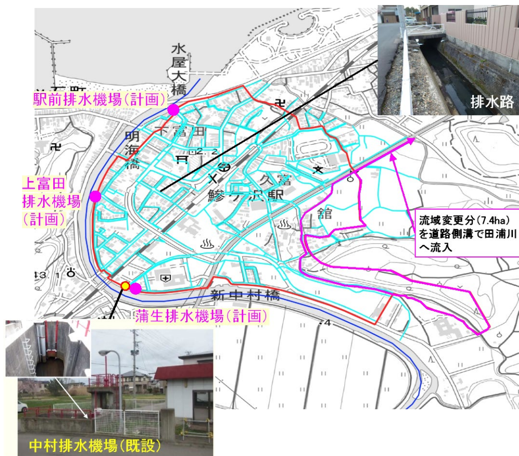
図 6-1 排水区域図
