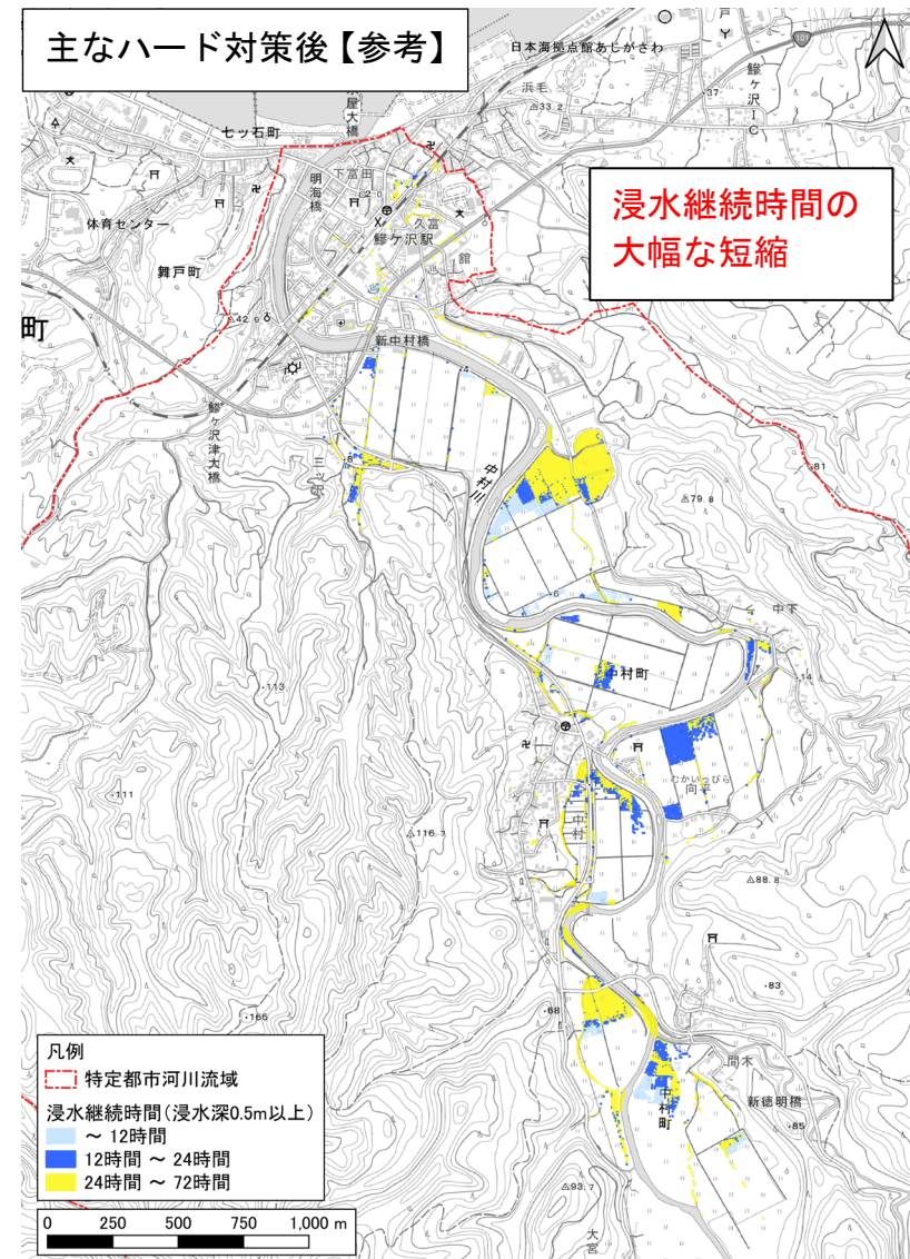
図 3-2 都市浸水想定浸水継続時間 (対策前と対策後の比較)
