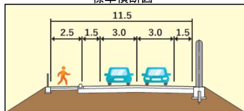
標準横断面図
