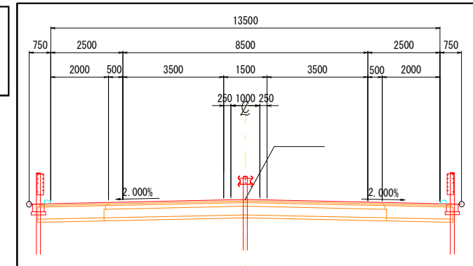
【標準横断図 (本線切土部)】
