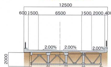
■標準断面図■
