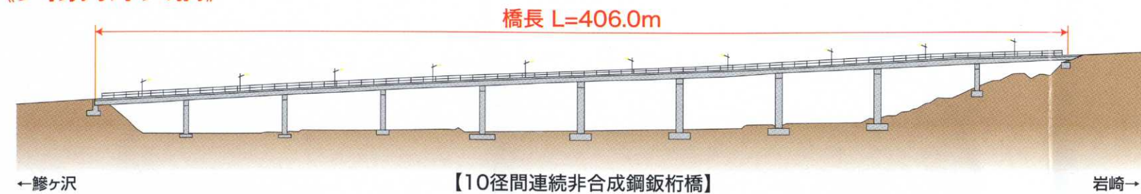
■側面図■
