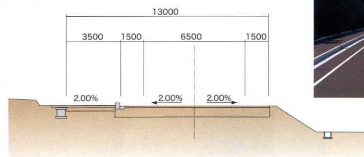
■標準断面図■
