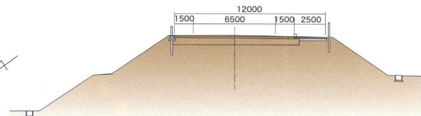
■標準断面図■
