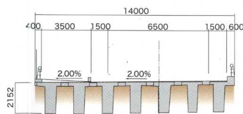
■標準断面図■
