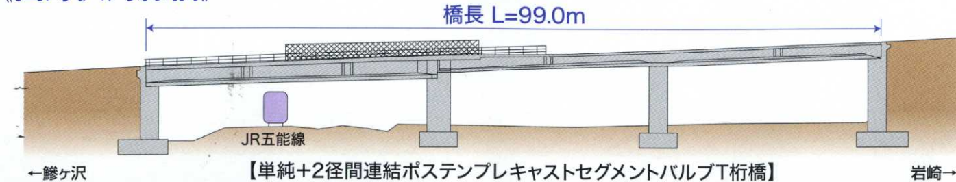
■側面図■
