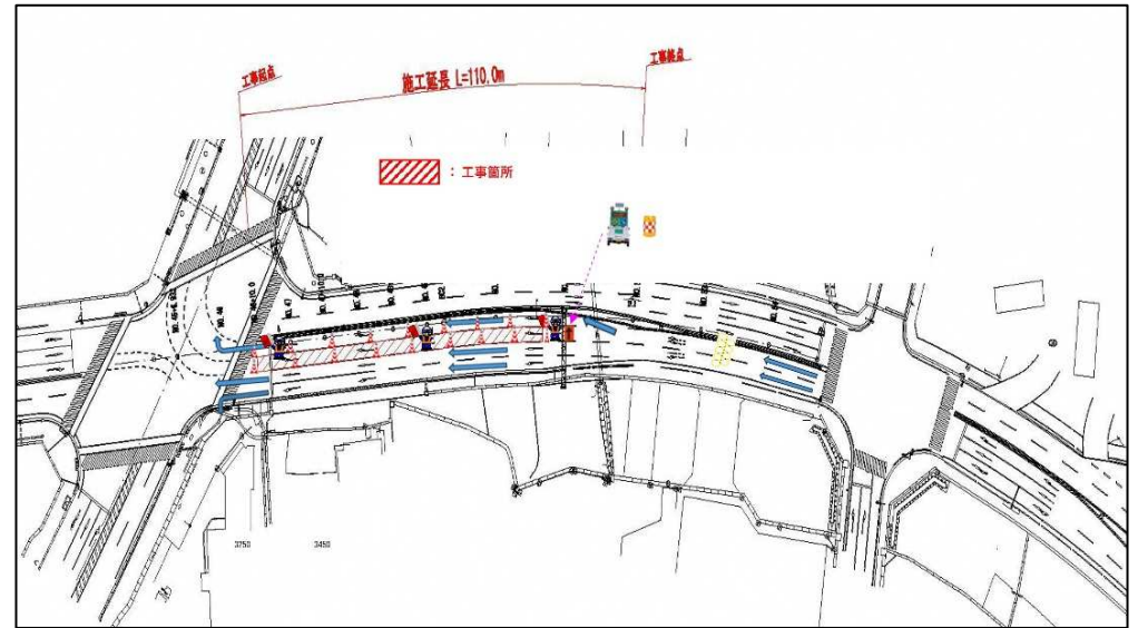
③ 11月6日（右折第2レーン→右折第1レーンを工事）
