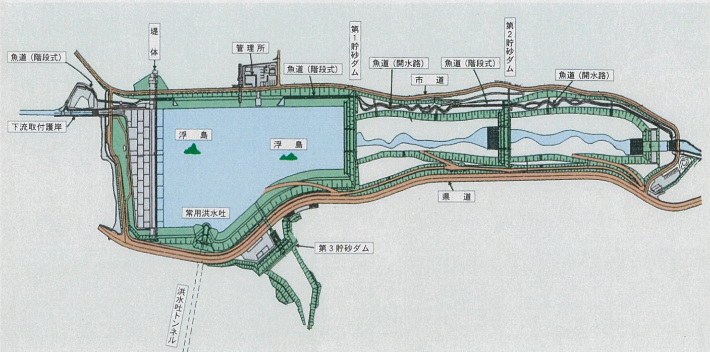
全体平面図
