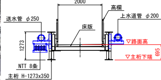
橋梁架替期間中のライフライン確保
