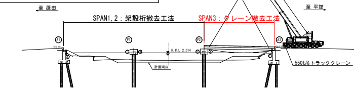
上部工撤去概略図
