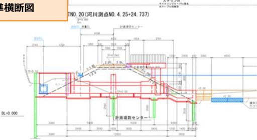
樋門標準横断面図
