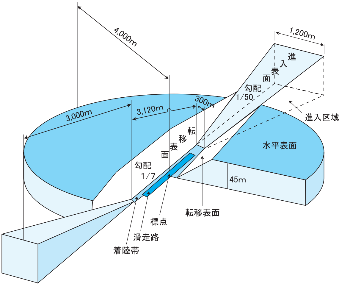
〈青森空港制限表面説明図〉
