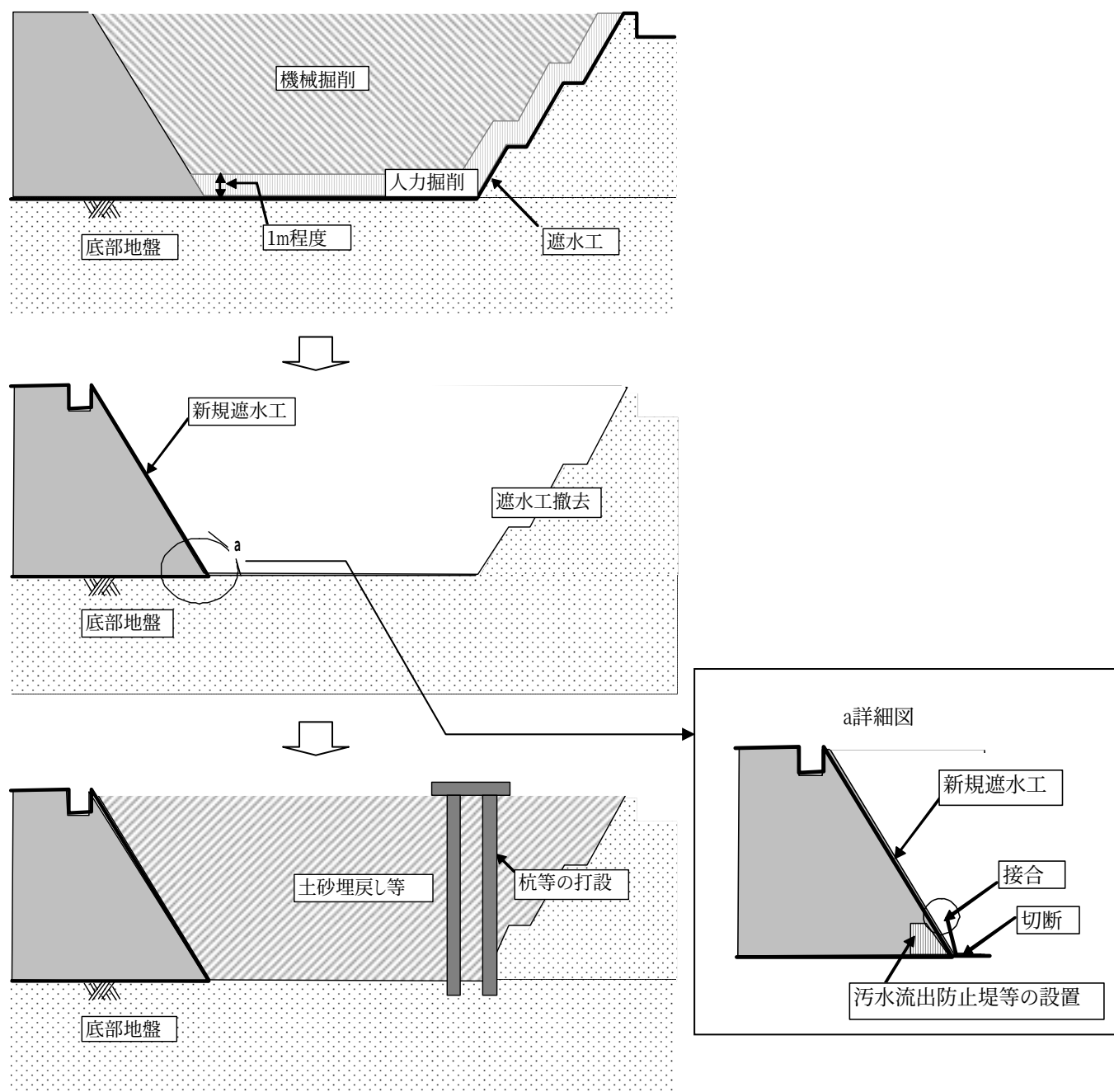
図 4-1 掘削による廃棄物・遮水シート除去と杭等の施工概念(オープン掘削)
