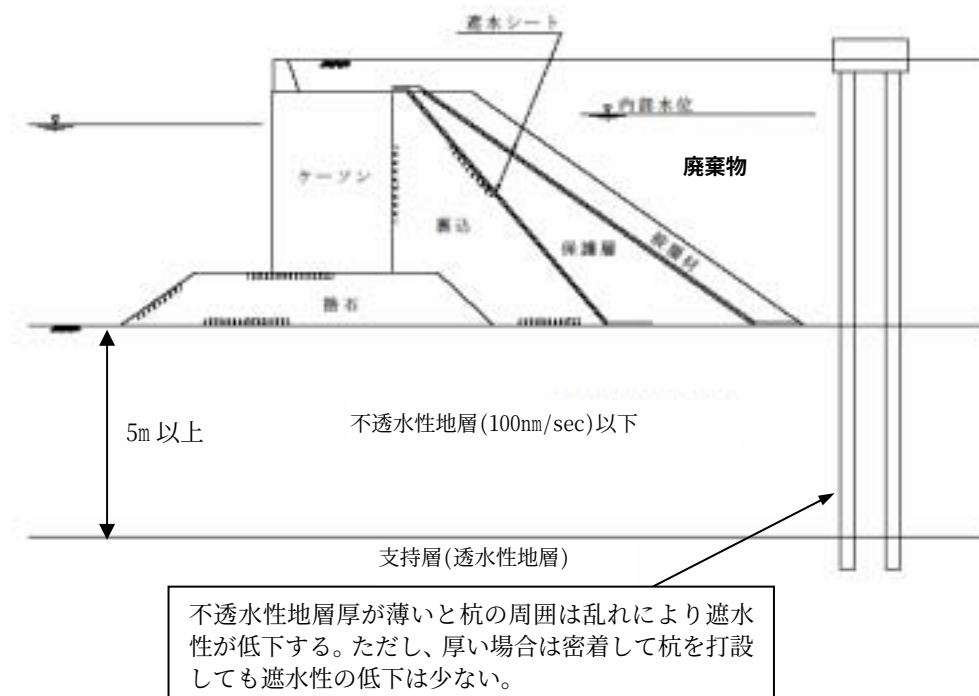
図 4-14 不透水性地層が 5\text{m} 未満となる場合の遮水工施工の概念
