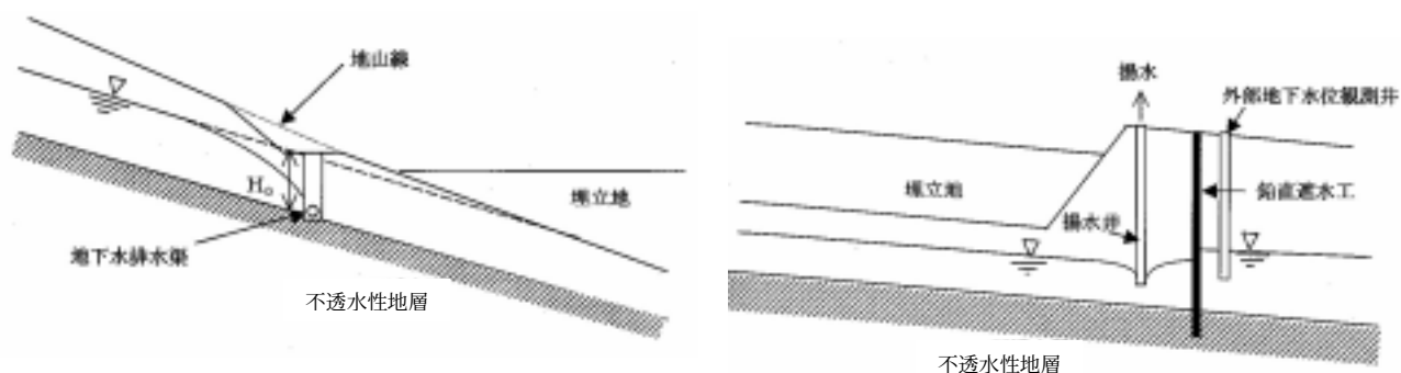
図 4-18 揚水による廃棄物埋立地上流部の地下水流入防止（左図）と鉛直遮水工と揚水井による汚染地下水の外部拡散防止（右図）の例 *5
