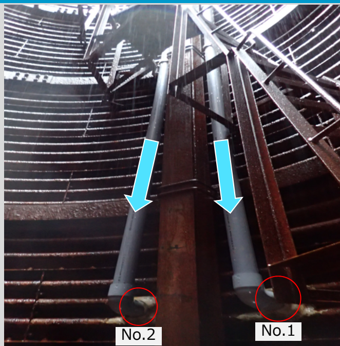
注水用横ボーリング R 3.8.19より注水開始
