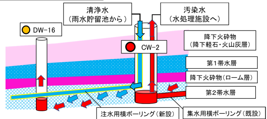
注水用横ボーリングの新設
