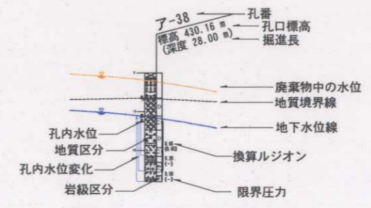
図-4 IV断面・VI断面 地質断面図
