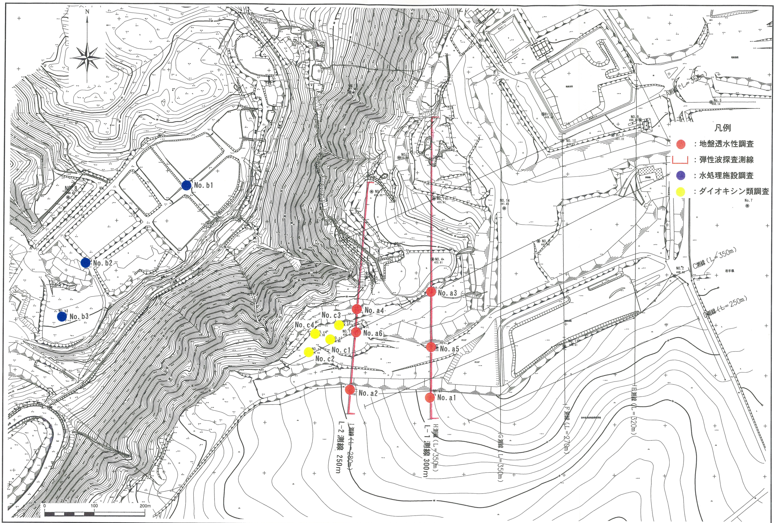
図 1. 3. 2 調査位置詳細図 (S=1/2,000)
