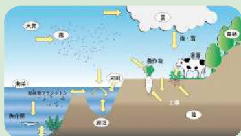
放射性物質の環境中での挙動をモデル化
