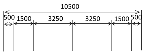
標準横断図（改良前）
