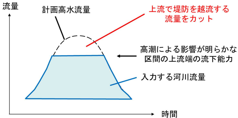
図-3 河川流量のピークカット
