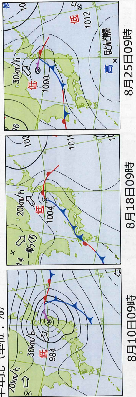
むつの気象経過図（令和3年8月1日～31日）
