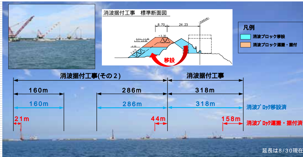
八戸港 北防波堤復旧状況 8/31現在(国土交通省資料)
