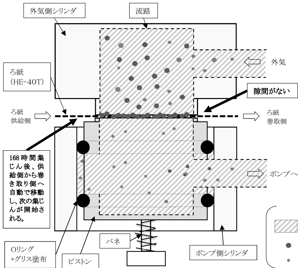
(a) 集じん部の概略(正常時)
