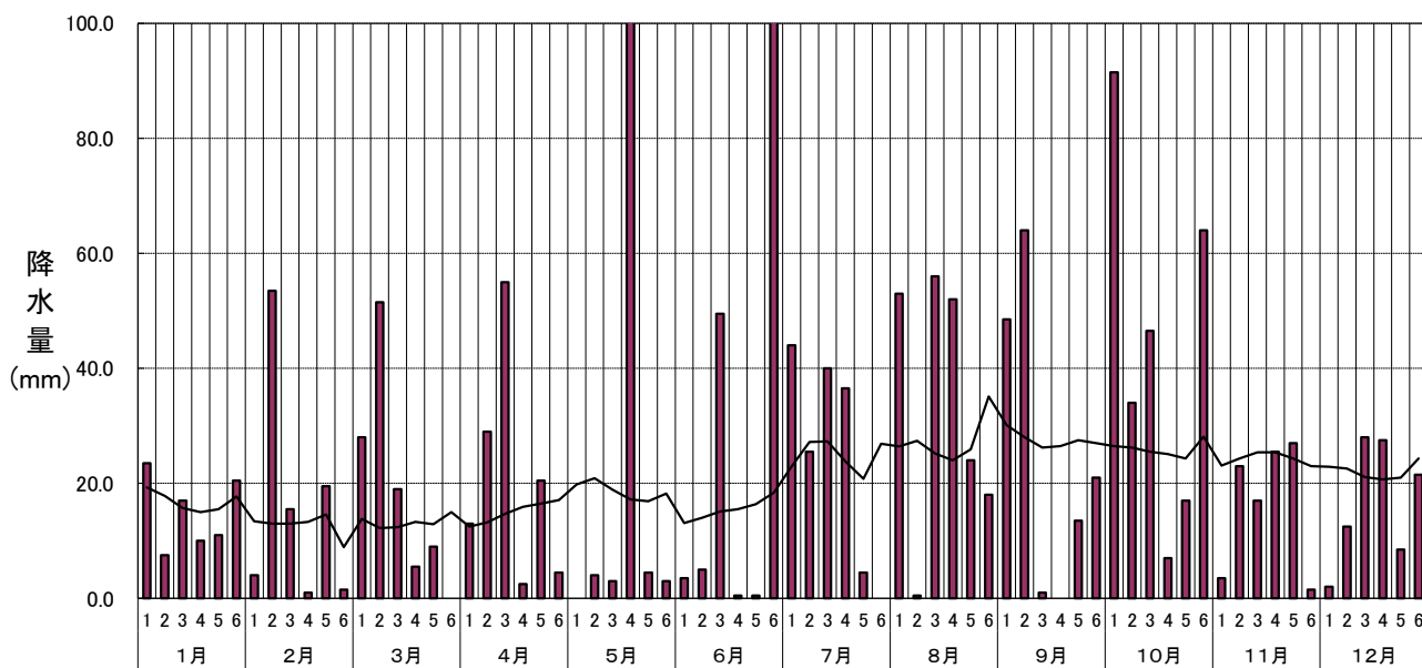
半旬別気象図 降水量(深浦:平成30年)
