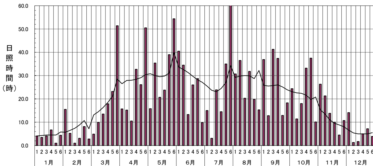
半旬別気象図 日照時間(深浦:平成30年)
