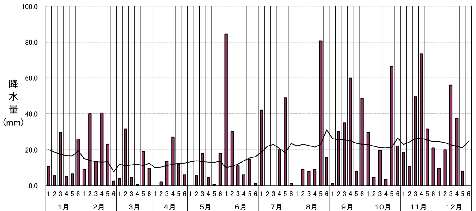
半旬別気象図 降水量(鱒ヶ沢:平成29年)
