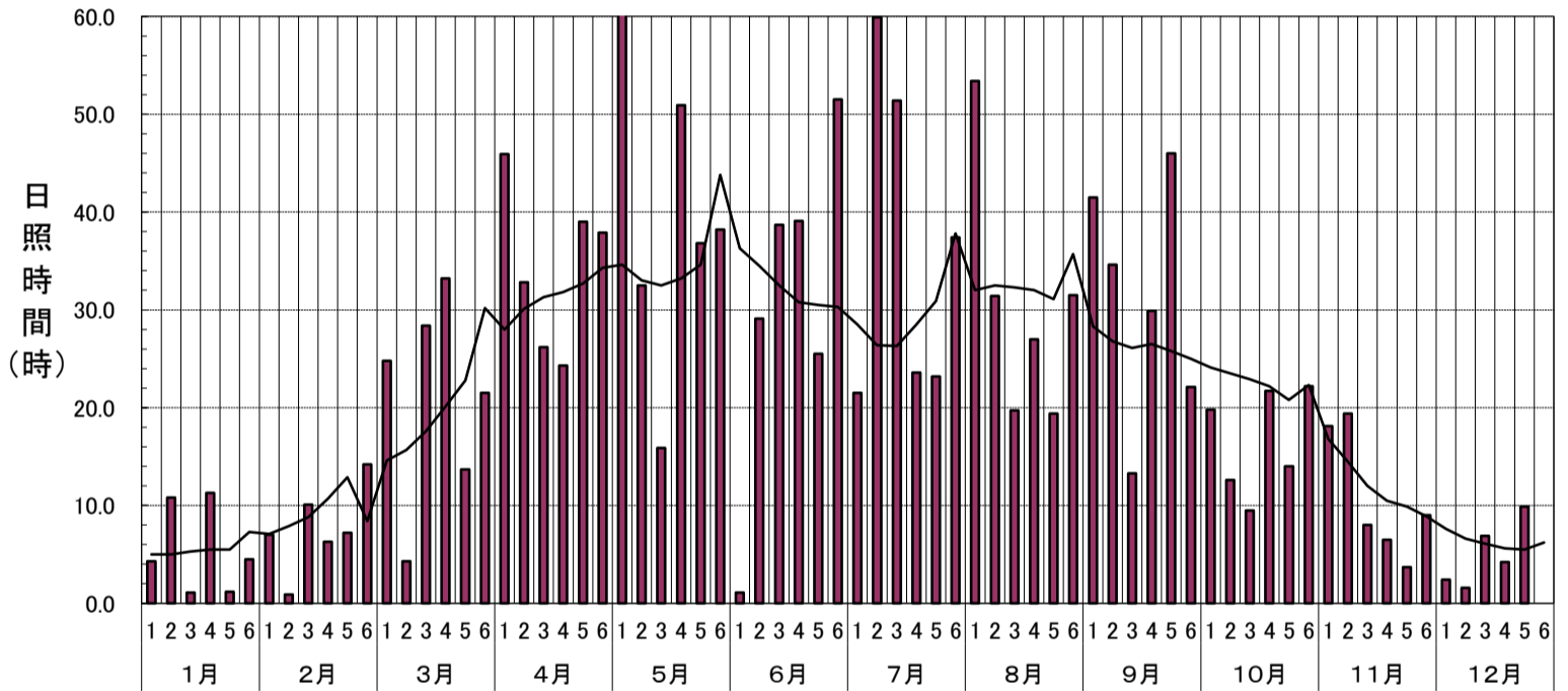
半旬別気象図 日照時間(鱒ヶ沢:平成29年)
