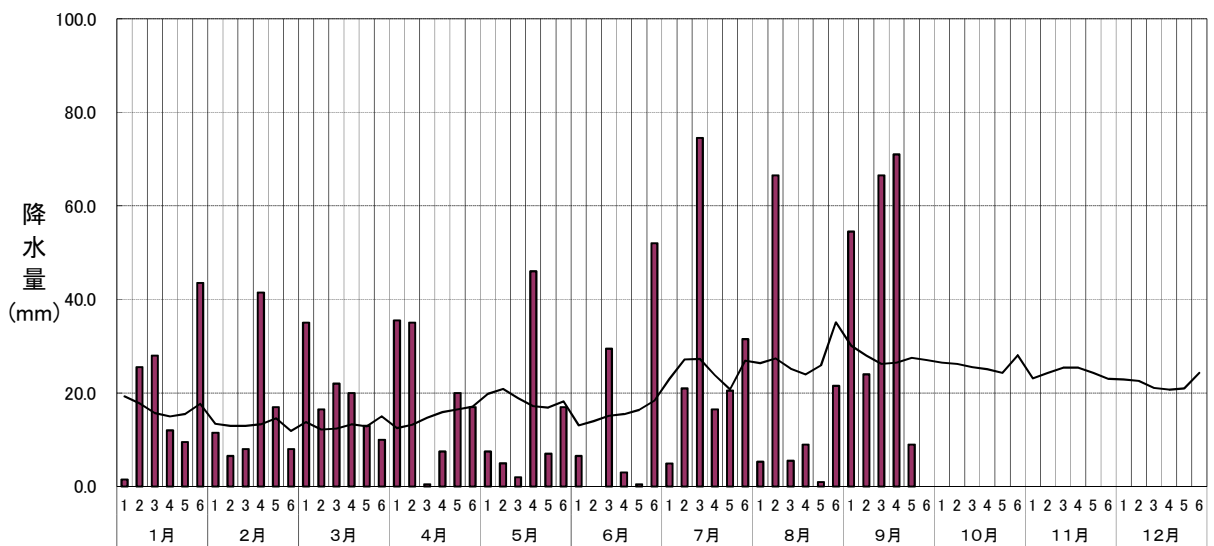
半旬別気象図 降水量(深浦:2020年)
