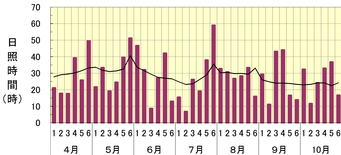
半旬別気象図・日照時間(弘前:平成30年)
