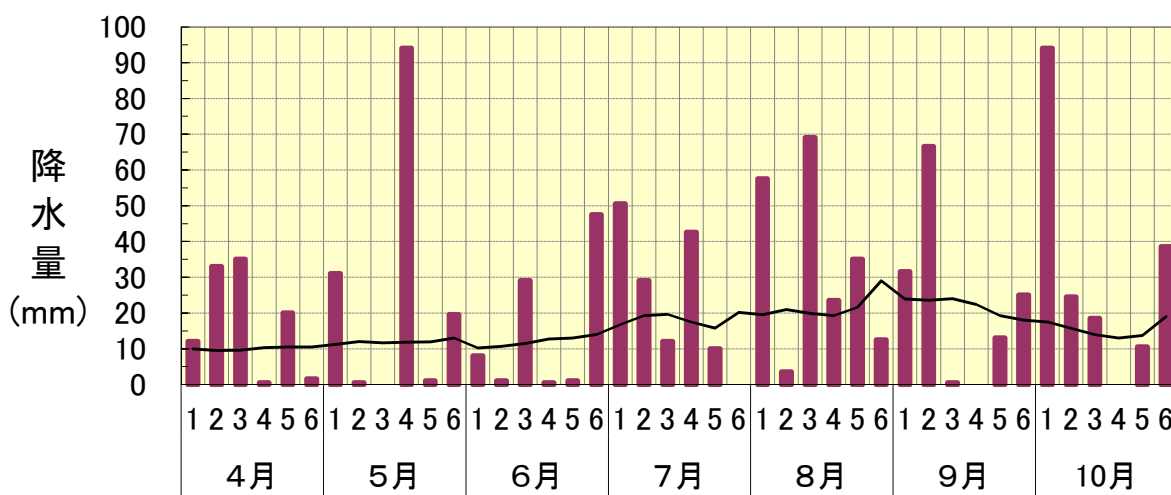
半旬別気象図・降水量(弘前:平成30年)
