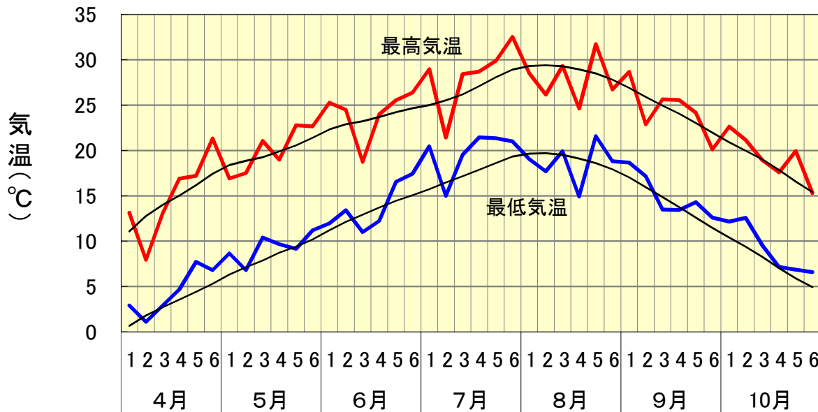
半旬別気象図 最高気温・最低気温(弘前:平成30年)
