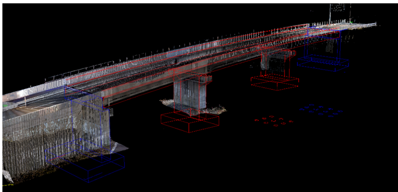
既存の竣工図データと3Dスキャナー調査との整合
