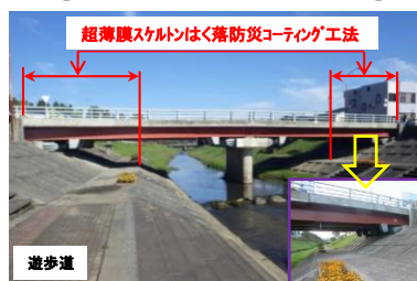
コンクリートのはく落防止対策(乙供橋)
