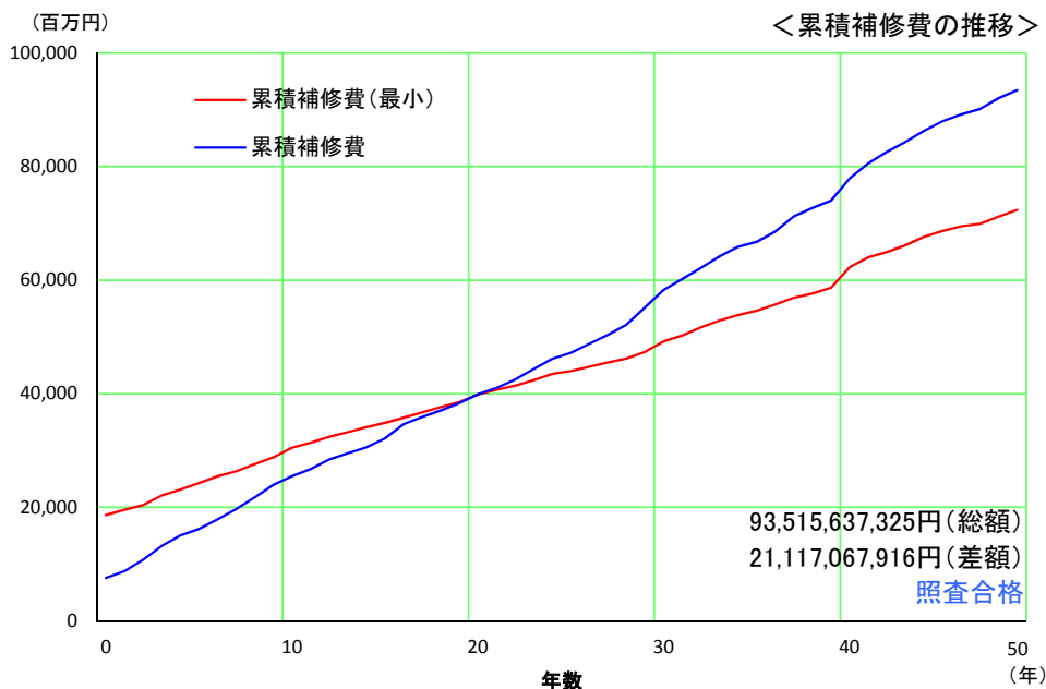
図 6-4 予算平準化前後の累計補修費の比較
