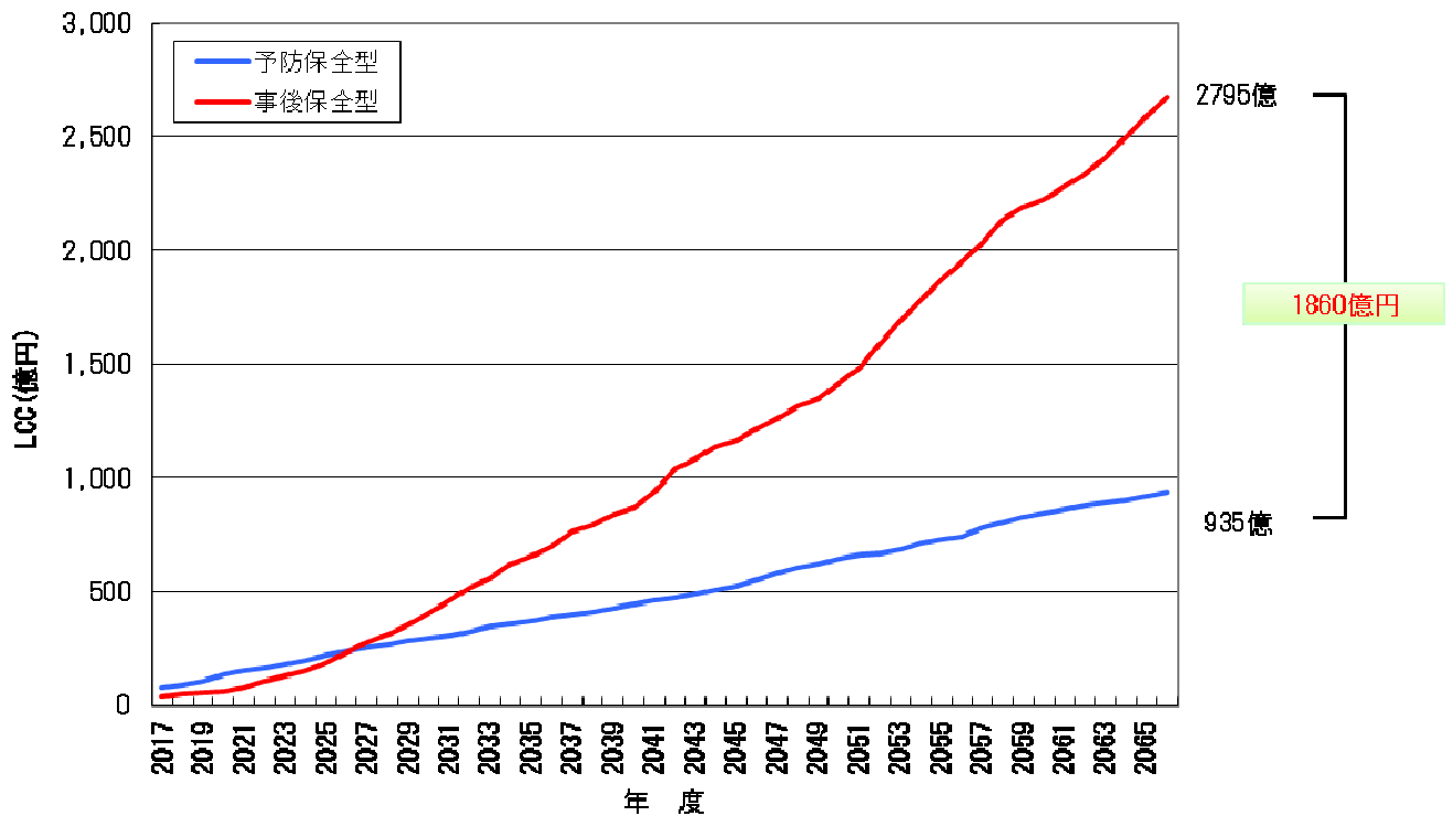
図 7-1 Aグループ橋梁のコスト削減効果
