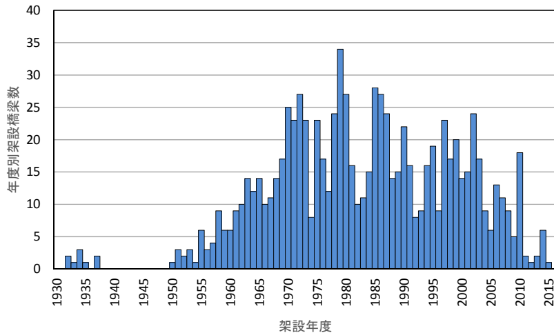
図 3-1 橋梁の架設年度の分布（橋長15m以上）
