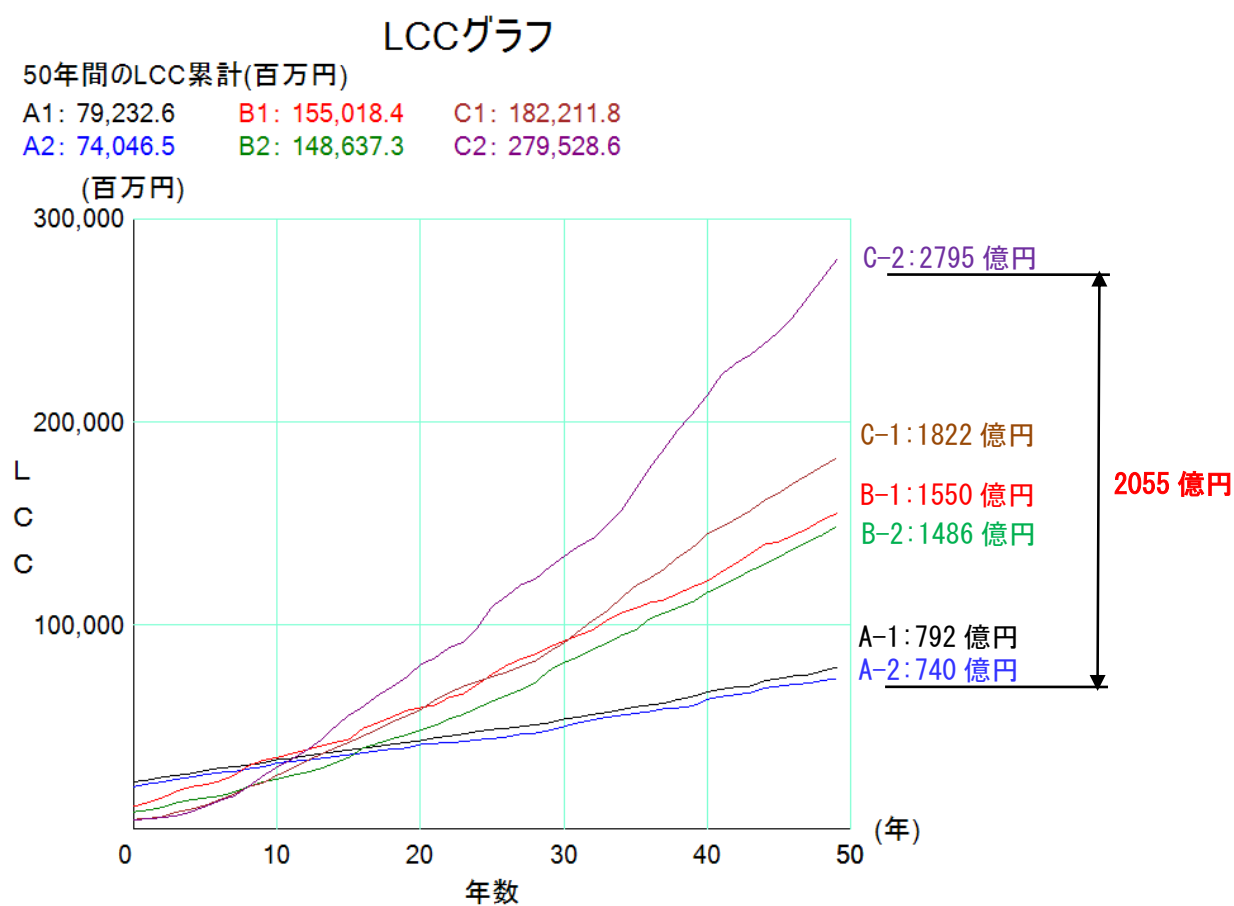
図 6-1 シナリオ別LCC算定結果
