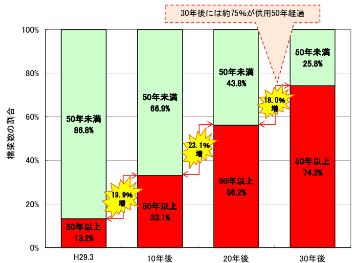
図 3-3 建設後経過年数別の割合（橋長15m以上）
