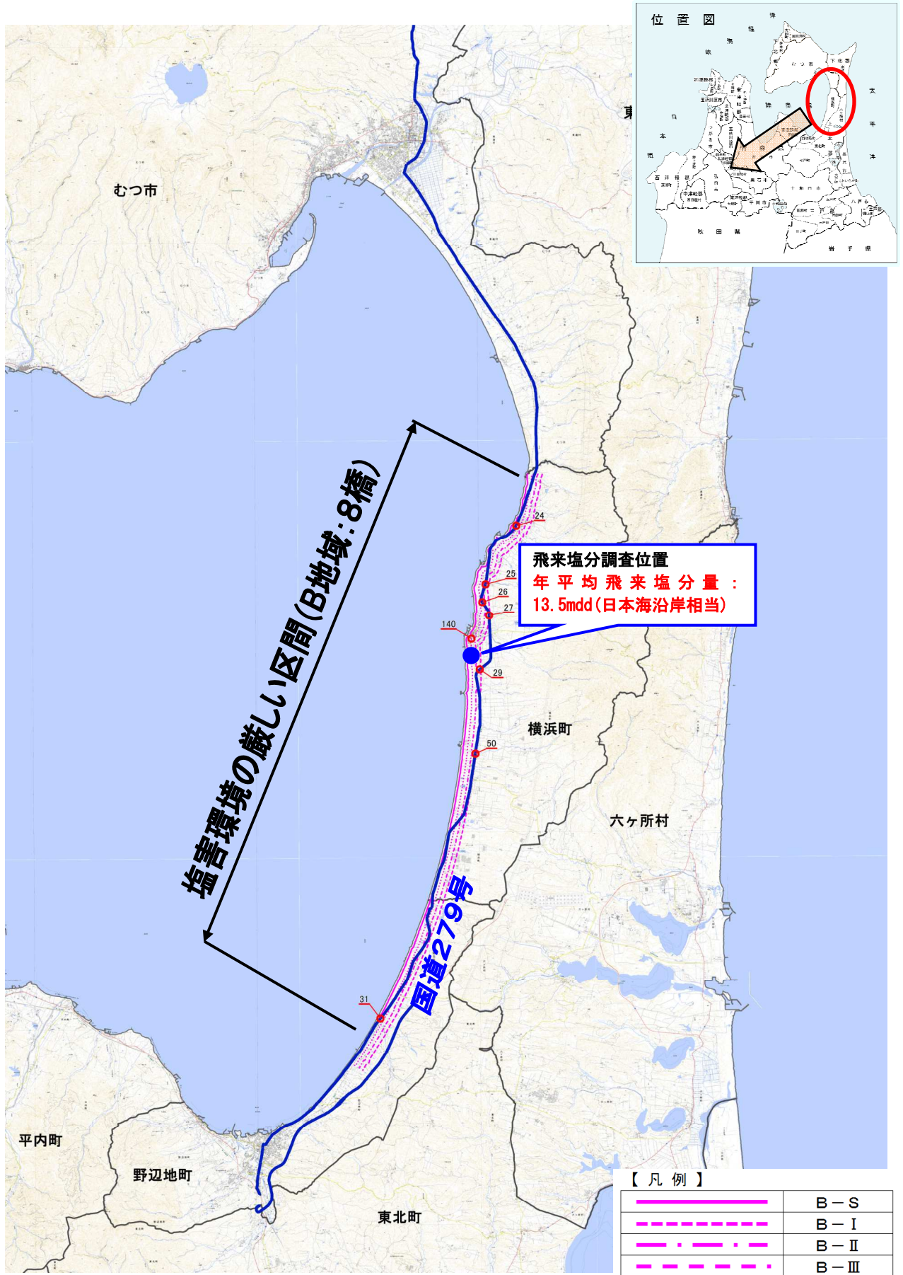
図 3-9 国道279号むつ湾沿岸塩害対策区分
