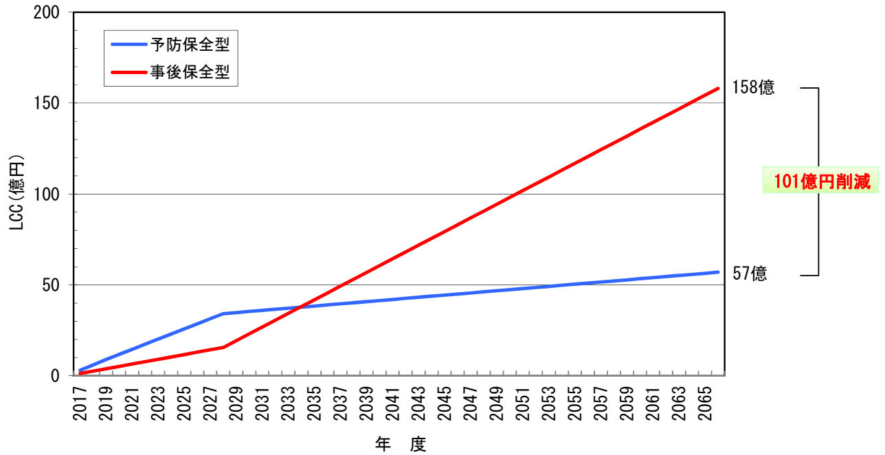
図 7-2 Bグループ橋梁のコスト縮減効果
