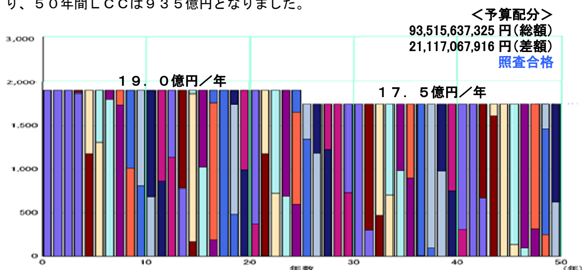
図 6-3 予算制約を考慮した予算平準化結果
