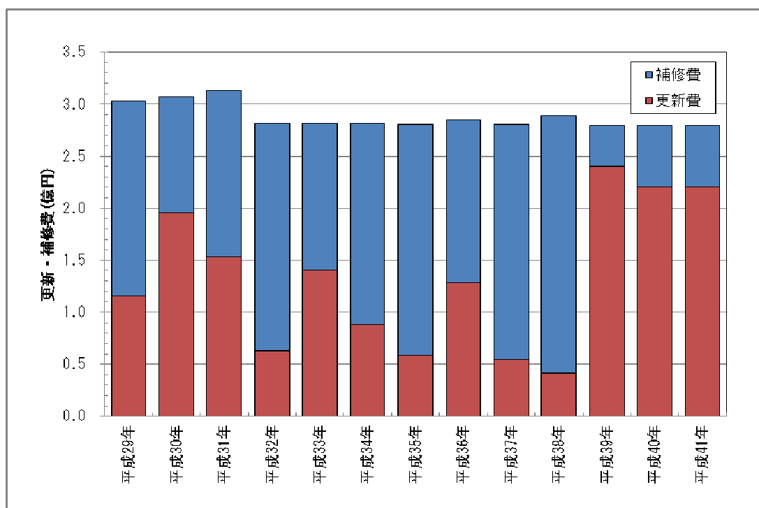
図 6-5 更新・補修費の推移 (13年間)
