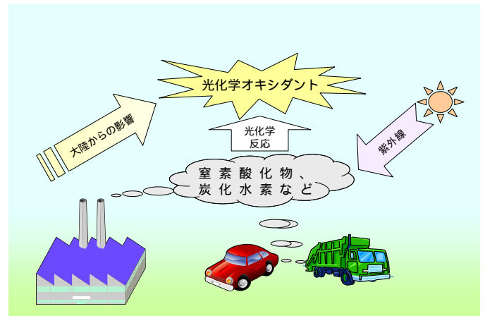
光化学オキシダント発生のしくみ
