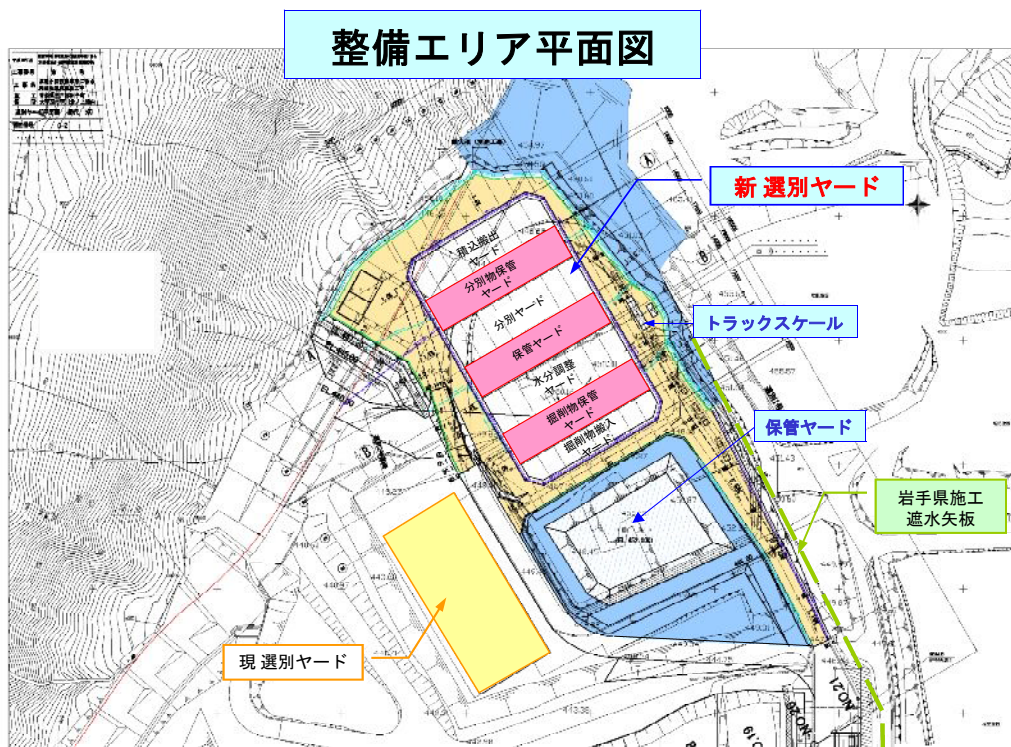
【新選別ヤード整備エリア平面図】
