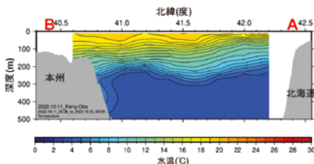
図5 フェリー航路上での水温観測結果 （令和4年10月）
