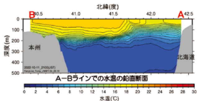
図4 シミュレーションでの水温分布計算結果 A-Bラインでの水温の鉛直断面（令和4年10月）
