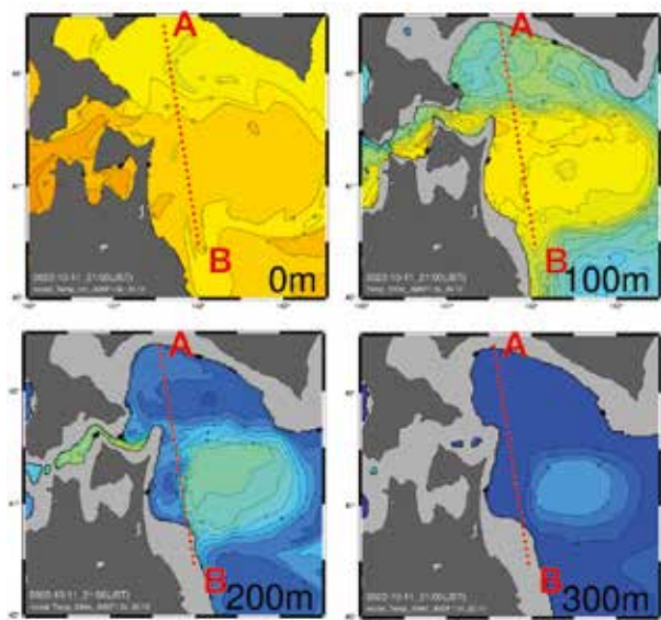
図3 シミュレーションによる水温分布計算結果 深度別の水温分布（令和4年10月）
